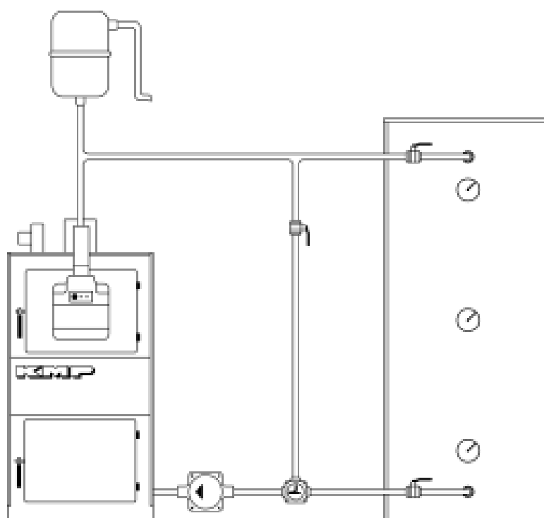
Fig. 5 Panna med ackumulatortank, principskiss.
