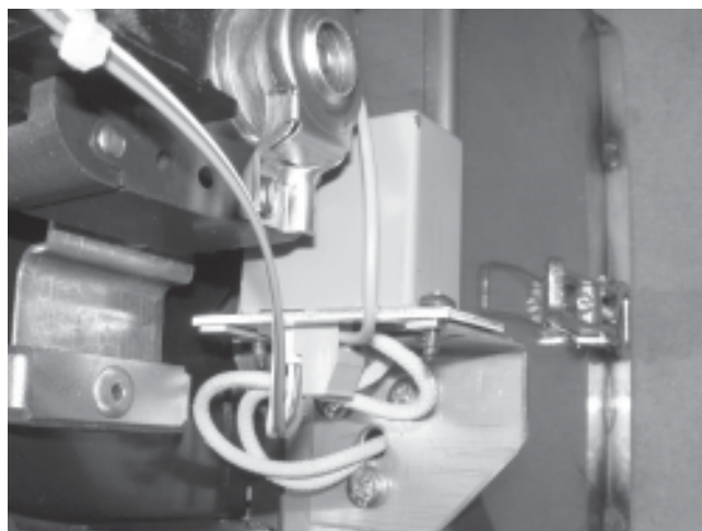
Fig. 6 Triacstyrning
