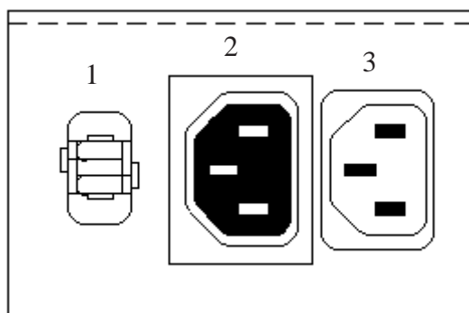
Fig. 2 Kontaktdon på brännaren.
